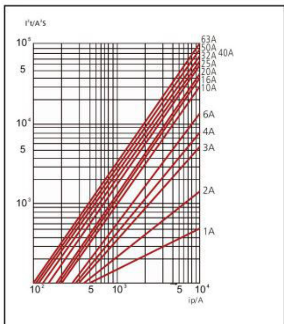
Durchlassenergie I^2t
